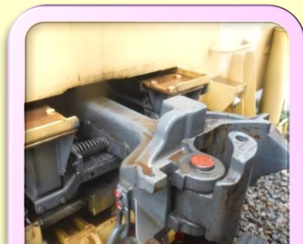
電力保守用車 連結器
